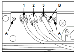
RYS. 18 (Wymiana termopary, pilota i wtyczki)
