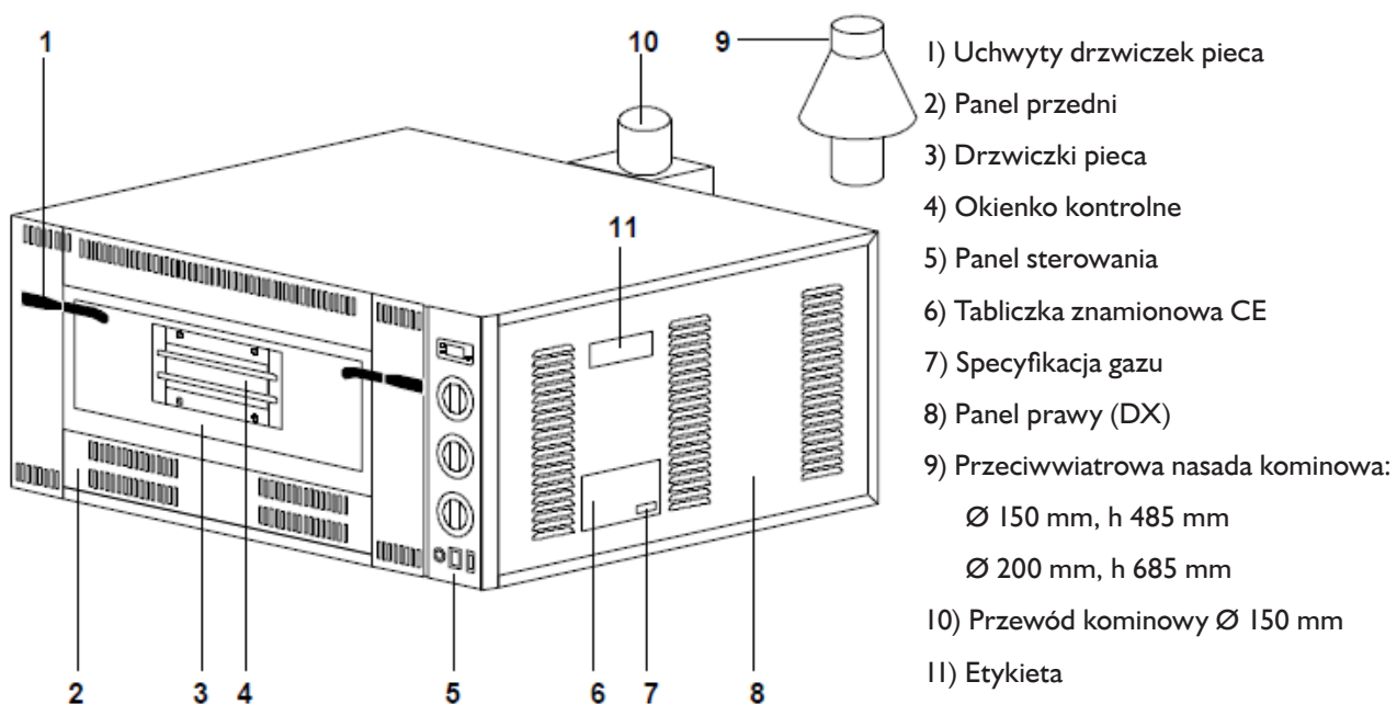
RYŚ. 3 (Wykaz elementów urządzenia)
