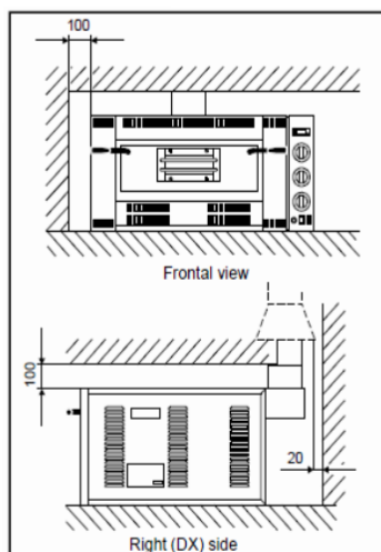
RYS. 5 (Minimalne odległości konieczne do zachowania przy ustawianiu urządzenia w miejscu instalacji)
