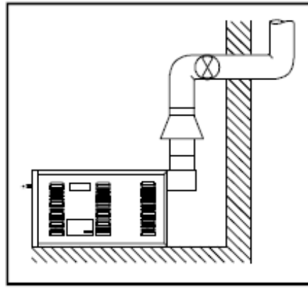
RYS. 12 (Odprowadzenie spalin z wykorzystaniem wentylatora wyciągowego)
