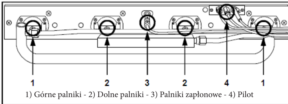
RYS. 8 (Wymiana palników: górnych, dolnych i zapłonowego)
