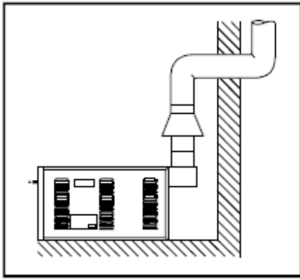
RYS. 11 (Grawitacyjne odprowadzenie spalin)
