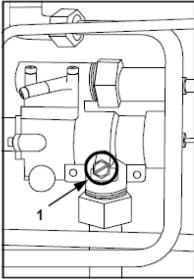
RYS. 7 (Kontrola ciśnienia gazu zasilającego)
