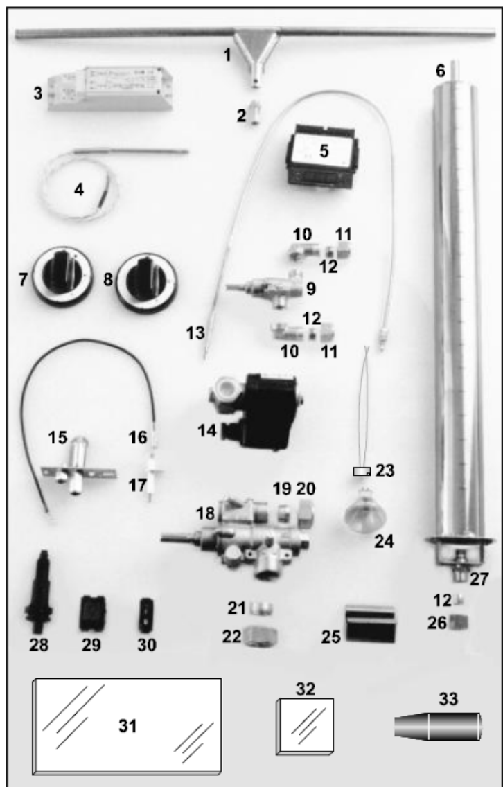
RYS. 20 (Części zamienne i elementy urządzenia)
