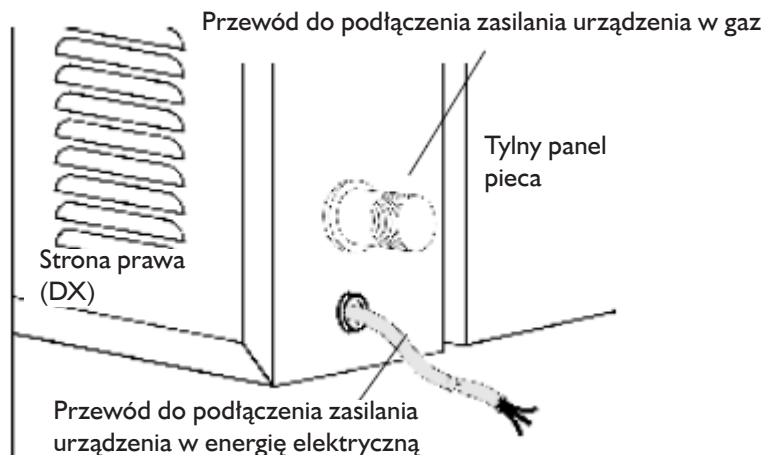
RYS. 6 (Podłączenie elektryczne i gazowe)
